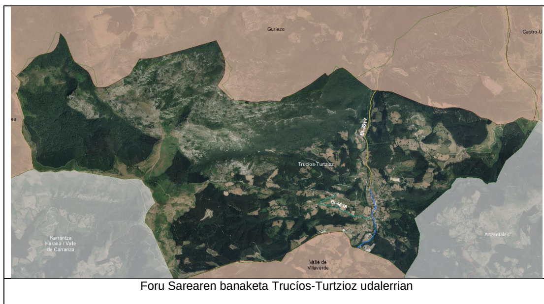
1. irudia. Trucíos-Turtzioz udalerrian zehar doazen errepideak.
